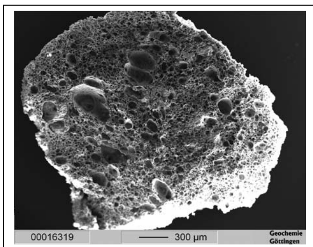
Abb3: REM-Bild (Sekundärelektronen) eines frisch gebrochenen Bims-Lapilli aus dem Herbstlabyrinth.
